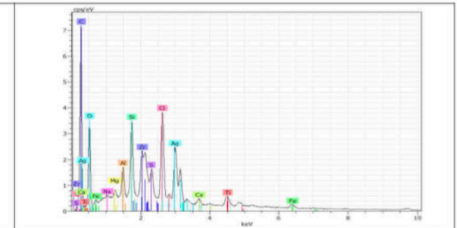
Espectro 1. Microanálisis de la zona analizada de Accesorio versión 8 / 23MA0068-1 zona 1.
