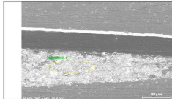
Imagen 6. Zona analizada de la muestra Accesorio versión 8 / 23MA0068-1 zona 1.
